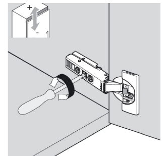
hoogteregeling - réglage en hauteur
