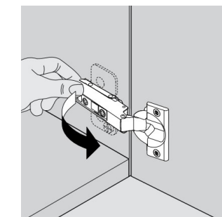
DEMONTAGE
