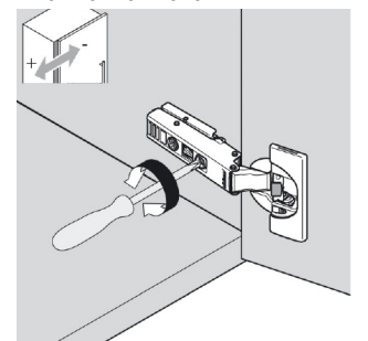
zijdelingse regeling - réglage latéral
