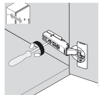
diepteregeling - réglage en profondeur
